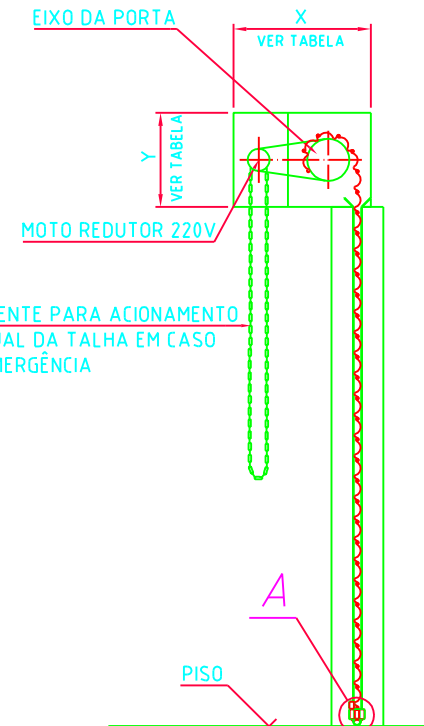
CORTE AA
